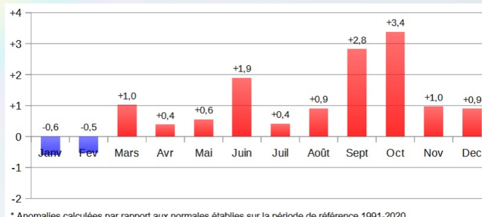
Figure 2: Anomalies* mensuelles de températures moyennes en ^{\circ}\text{C} pour l'année 2023 sur la commune de Seysses-Savès.
