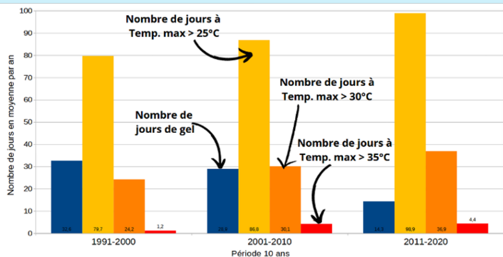
Figure 2: Evolution par période de 10 ans du nombre de jours moyen annuel de gel et de températures maximales >25° C, >30° C et >35° C
