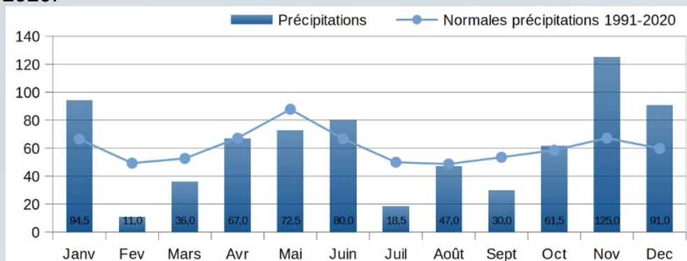
Figure 1: Hauteurs mensuelles de précipitations (barres) comparées aux normales climatologiques (points) pour l'année 2023 sur la commune de Seysses-Savès.
