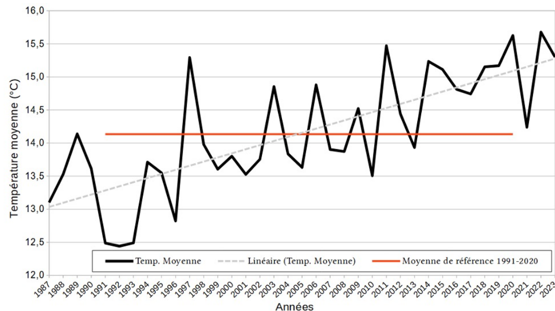
Figure 1: Evolution de la température moyenne (trait noir) sur la commune de Seysses-Savès entre 1987 et 2023. Sont indiquées aussi la moyenne sur la période de référence 1991-2020 (trait rouge) et la tendance linéaire (pointillés gris).
